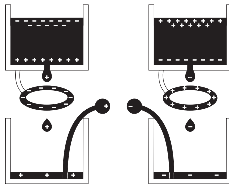
Рис. 7.40: Начальная фаза работы генератора Кельвина.
