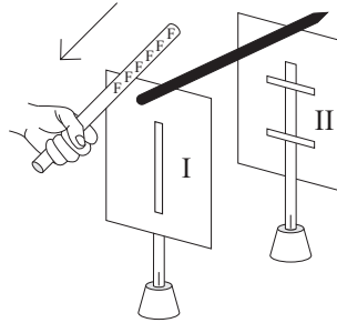
Рис. 6.19: Два первоначально разряженных электроскопа соединены деревянным шампуром. Электризованная солома царапает по электроскопу I .
