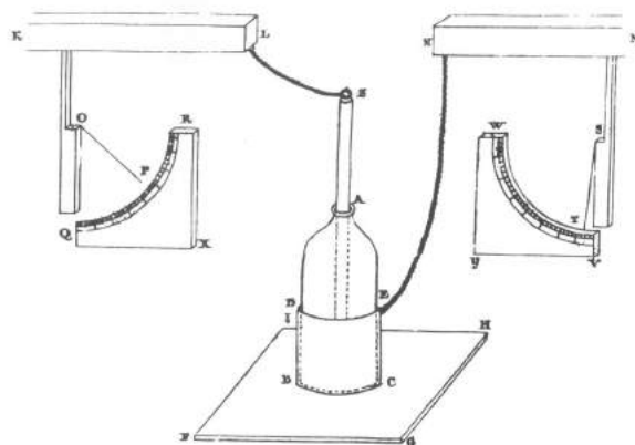
Рис. 6.40: Электromетры Рихмана, подсоединенные к лейденской банке. Каждый из электрометров имеет одиночную подвижную полосу.
