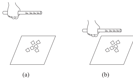
Рис. 7.43: натертая солома теряет свой заряд спустя несколько часов после первоначального трения. Она больше не притягивает лежащие рядом с ней небольшие кусочки бумаги.
