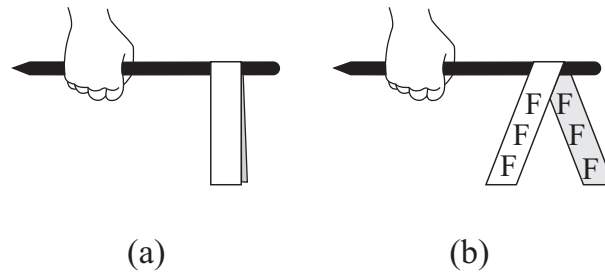
Рис. 4.1: (a) Нейтральная пластиковая полоса свисает вертикально с горизонтальной деревянной шпаги. (b) Отталкивание между двумя половинами натертой пластиковой полоски.
