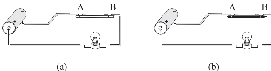
Рис. 6.27: (a) Лампочка не включается при соединении A и B пластиковой соломой. (b) Лампочка не загорается и при соединении A и B посредством деревянного шпajка.
