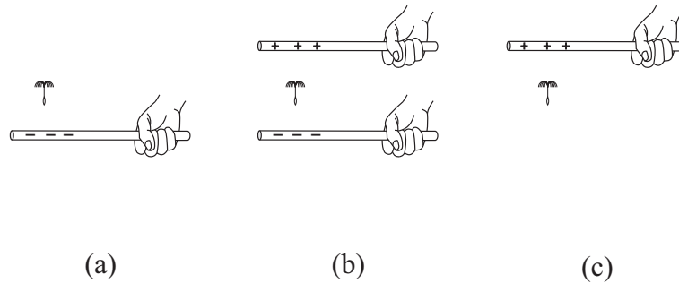
Рис. 5.22: (a) Отрицательный одуванчик, парящий над отрицательной соломой. (b) Отрицательный одуванчик, парящий между отрицательной и положительной соломой. (c) Отрицательный одуванчик, парящий под положительной соломой.
