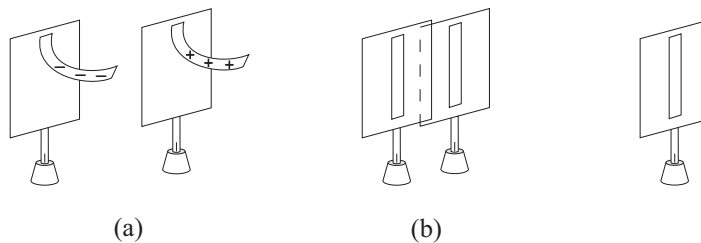
Рис. 6.30: (a) Положительный электроскоп и отрицательный электроскоп. (b) После контакта полоски падают. (c) После разделения полоски остаются в вертикальном положении, указывая на то, что электроскопы теперь разряжены.
