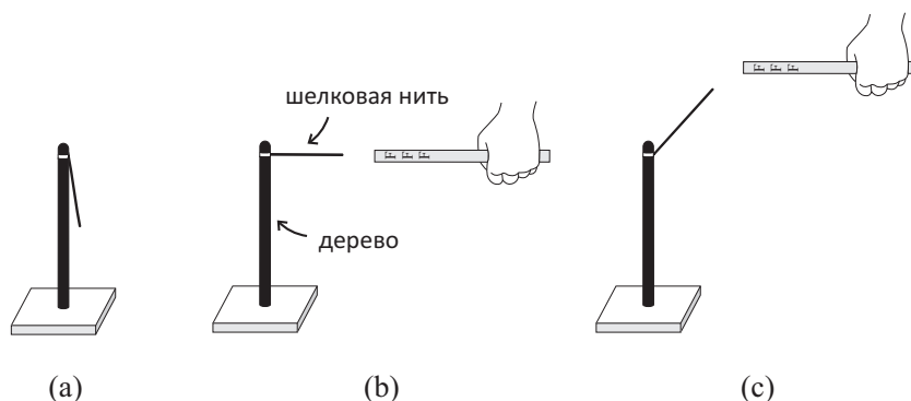
Рис. 7.27: Грей притягивает шелковую нить, поместив кусок натертой бумаги около нее.
