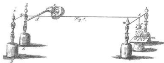
Рис. В.11: натертая стеклянная трубка касается горизонтальной веревки и шар притягивает легкие тела. Вербка поддерживается изолирующими струнами.
