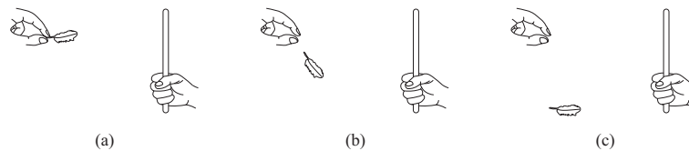
Рис. 4.9: Пуховое перо освобождается вблизи ненатертой стеклянной трубки. Оно падает на землю.
