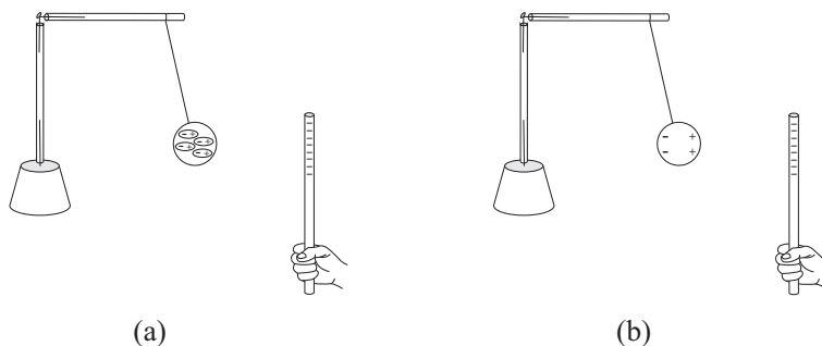
Рис. 8.1: (а) натертый пластик поляризует и притягивает пластиковый диск. (b) Эффективная поляризация пластикового диска.
