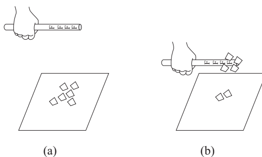
Рис. 2.3: (а) натертая солома находится далеко от мелких кусков бумаги. (б) натертая солома притягивает бумажки на близком расстоянии.
