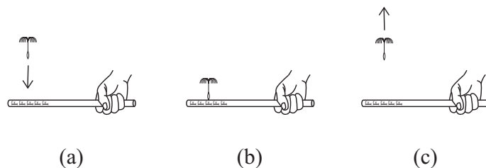
Рис. 4.5: Эксперимент 4.4 легко проводить с одуванчиком, плавающим над натертой волосами пластиковой соломой.
