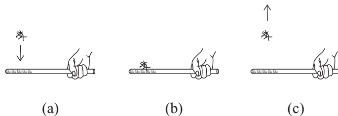
Рис. 4.4: (а) Кусок хлопка вначале притягивается натертой пластиковой соломой. (б) Хлопок касается натертой части соломой. (с) После контакта хлопок отталкивается от соломой. Затем его можно держать в парящем состоянии над соломой, несмотря на гравитационное притяжение Земли!
