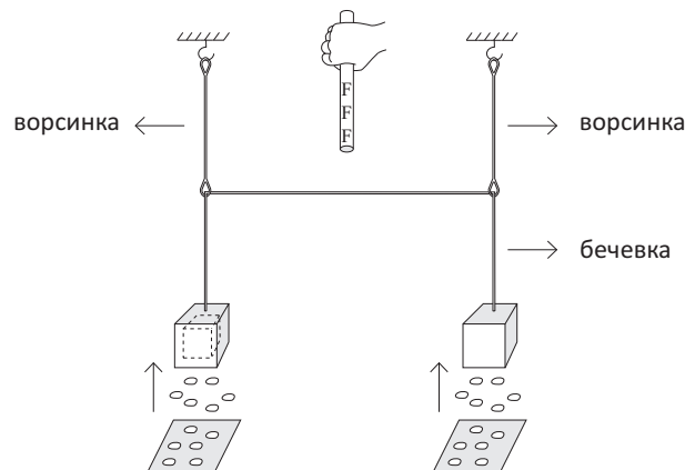
Рис. В.21: Полый куб и сплошной куб притягивают с одинаковой силой.
