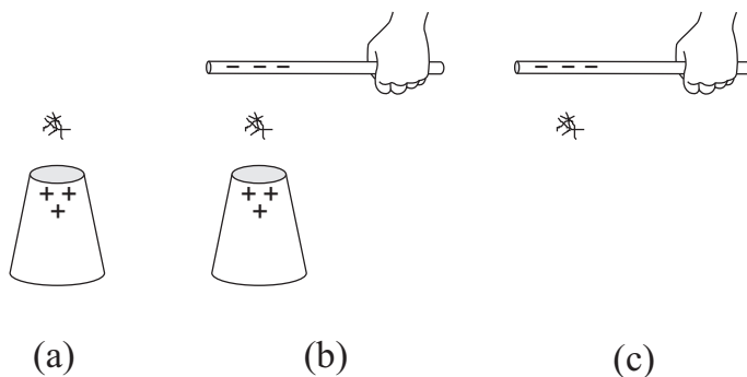
Рис. 5.12: (а) Положительный кусок хлопка можно поддерживать в парящем над положительным стеклом состоянии. (b) Он также может плавать между положительным стеклом снизу и отрицательной соломой сверху. (с) Мы можем удалить стекло и парить кусочек хлопка под отрицательной соломой.
