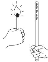
Рис. 7.44: Мы зажигаем спичку возле натертой соломы.
