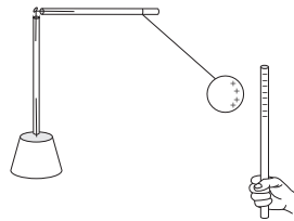
Рис. 8.3: Наэлектризованный бумажный диск притягивается натертой соломой.
