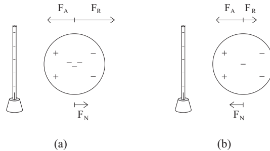
Рис. 7.33: (a) При значительном суммарном заряде на проводнике, суммарная отталкивающая сила сохранится между ним и отрицательным изолятором. (b) Если проводник имеет лишь небольшой суммарный заряд, сила притяжения, связанная с его поляризацией, будет превышать силу отталкивания, обусловленную наличием суммарного заряда, что дает в итоге притягивающую силу.
