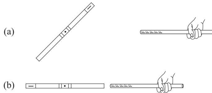
Рис. 5.23: Отрицательно заряженная алюминиевая фольга версориума Дюфе отталкивается приближающимся к ней наэлектризованным телом.
