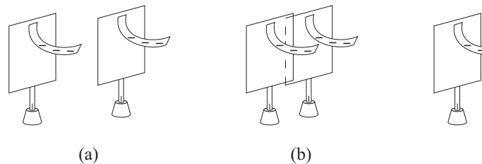
Рис. 6.29: (а) Два электроскопа, наэлектризованные зарядами одного знака. (b) Картоны касаются друг друга, но ничего не происходит. (с) После разделения, полосы остаются в поднятом состоянии.
