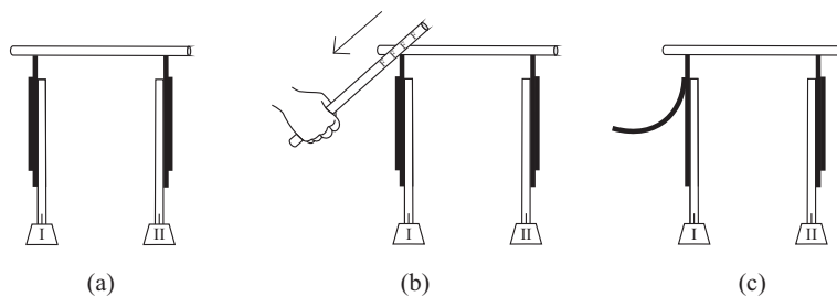
Рис. 6.18: (а) Два первоначально заряженных электроскопа соединены нейтральной соломой. (b) Вторая электризованная солома царапает по верхнему краю электроскопа I . (с) Заряженная солома удаляется. Мы видим, что только полоска электроскопа I поднимается.
