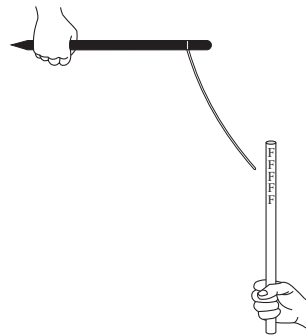
Рис. 4.29: Притяжение маятниковой нити натертым пластиком.
