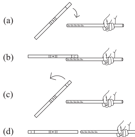
Рис. 4.24: (а) Алюминиевая фольга изначально притягивается натертым пластиком. (б) Алюминиевая фольга соприкасается с натертым участком соломы. (с) После контакта, алюминиевая фольга отталкивается от соломы. (d) Конечная равновесная ориентация версориума.
