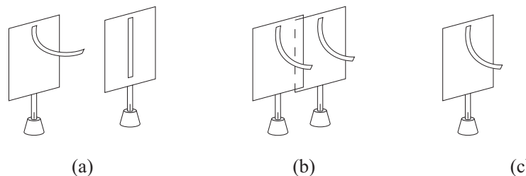
Рис. 6.31: (а) Заряженный и незаряженный электрометры. (б) Контакт между картонами. (с) Разъединение после контакта. Полосы остаются в поднятом состоянии, но с меньшим по сравнению с (а) углом наклона.
