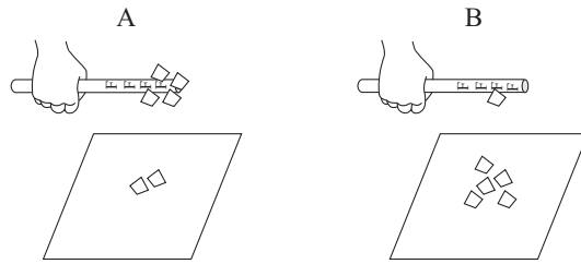
Рис. 5.28: Соломки A и B находятся на одинаковом расстоянии от стола. Мы заключаем, что солома A наэлектризована в большей степени, чем B , поскольку она притягивает больше кусочков бумаги.
