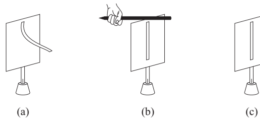
Рис. 6.14: (a) Изначально заряженный электроскоп. (b) Мы держим один конец деревянного шпажка в руке и трогаем верхний край электроскопа другим концом шпажка. Полоса сразу падает. (c) При удалении шпажка, полоса остается внизу. То есть электризованный электроскоп разряжается, когда мы касаемся его деревянным предметом в наших руках.
