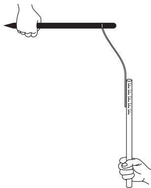
Рис. 4.30: Подвесная нить Грея прилипает к натертому пластику после контакта.
