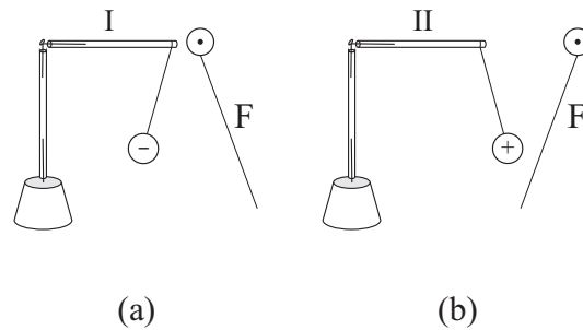
Рис. 5.21: Процедура Дюфе для обнаружения знака заряда наэлектризованного тела. В этом примере натертый пластик отталкивается отрицательно заряженным маятником, (a), и притягивается положительно заряженным маятником, (b). Таким образом, мы приходим к выводу, что пластик отрицательно заряжен.
