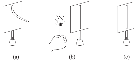
Рис. 7.42: (а) Электризованный электроскоп. (b) Полоса падает в течение нескольких секунд, если зажечь спичку или зажигалку в ее окрестности. (с) После удаления спички, полоса остается в висячем положении.
