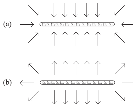
Рис. 4.34: (a) Стрелки, которые еще не прикоснулись к натертой соломе, притягиваются к ней. (b) После контакта они отталкиваются от нее.
