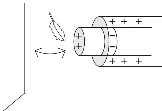
Рис. В.4: Поляризация проводящей пробки под действием натертого стекла. Проводящее перо притягивается распределенными по внешней поверхности пробки зарядами.
