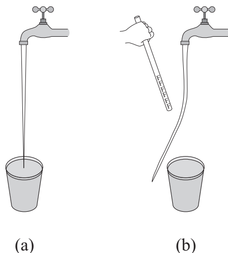
Рис. 2.6: Натертая солома притягивает поток воды.
