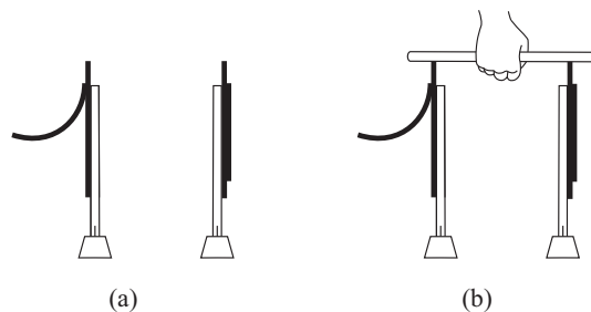
Рис. 6.32: (а) Электроскоп I заряжается. (б) Нейтральная солома размещается таким образом, чтобы соединить электроскопы. Ничего при этом не происходит.
