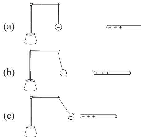
Рис. 5.26: Уменьшая расстояние между отрицательным бумажным диском и положительным кончиком натертой соломой, мы увеличиваем силу притяжения между ними.
