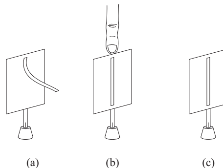
Рис. 6.6: Разрядка электроскопа посредством его касания. (a) Первоначально заряженный электроскоп. (b) Когда мы трогаем верхний край картона, полоска падает. (c) Полоса остается в вертикальном положении после удаления пальца.
