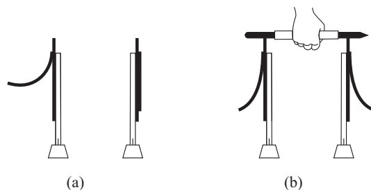
Рис. 6.33: (а) Заряжен только электроскоп I . (б) Деревянный шпатель окружен пластиковой соломой и покоится на двух электроскопах. Заметим, что полоса I немного падает, в то время как полоса II слегка поднимается.
