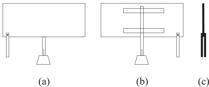
Рис. 6.3: (а) Классический электроскоп с лицевой стороны. (б) Вид сзади. (с) Вид сбоку, с изображением лишь тонкого картона и двух полос.
