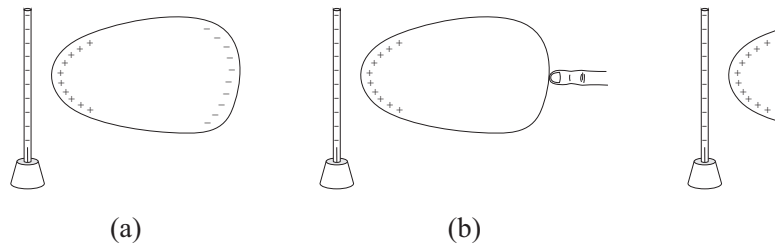
Рис. 7.30: Заземление проводника в присутствии поблизости заряженного тела.
