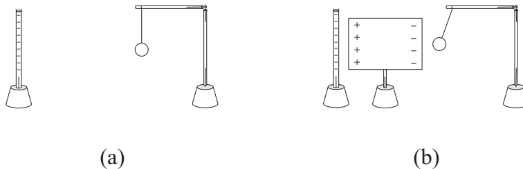
Рис. 7.13: (a) Отрицательная солома на расстоянии 15 см от нейтрального маятника. (b) Когда мы помещаем проводящую пластину между ними, мы наблюдаем притяжение маятника пластиной.
