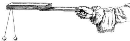
Рис. 6.38: Электроскоп Кантона.
