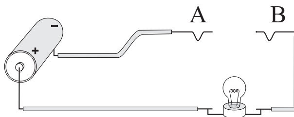
Рис. 6.25: Тестер цепи.
