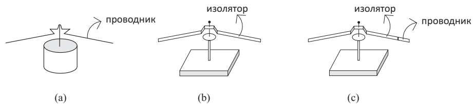
Рис. 6.21: Компоненты версориума. (a) Металлический версориум. (b) Пластиковый версориум. (c) Версориум Дюфе.
