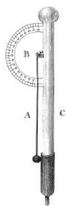
Рис. 6.41: Электрометр Хенли.
