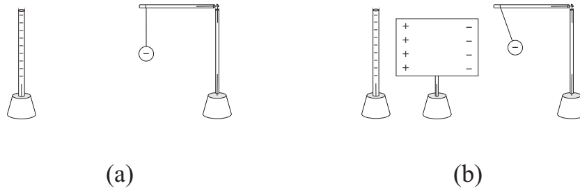
Рис. 7.14: (а) Отрицательно заряженная солома не оказывает заметного влияния на отрицательно заряженный маятник, который находится далеко от нее. (b) Если поместить нейтральный прямоугольный проводник между ними, возникает отталкивание.
