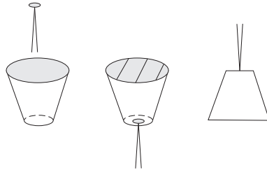
Рис. 4.14: Опора электрического маятника, изготовленная из тонкого пластикового стаканчика для кофе, бумажной крепежки и гипсового теста.
