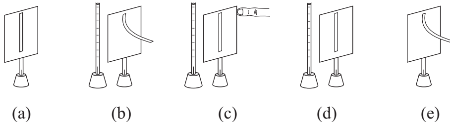
Рис. 7.18: Вторая схема для зарядки электроскопа по индукции.
