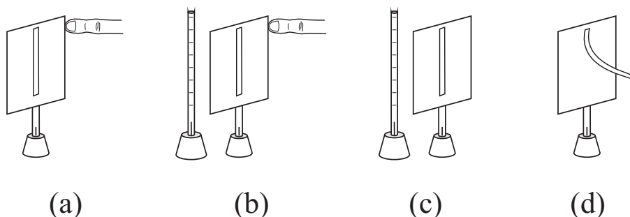
Рис. 7.21: Третья схема индукционной зарядки электроскопа.
