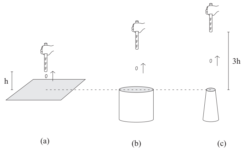
Рис. В.22: (а) Маленький листик латуни притягивается на высоте H от начального положения на полу. (b) Он поднимается еще выше, когда лежит на столе или на проводящем цилиндре 30 см в диаметре. (с) Когда он лежит на коническом проводнике, он притягивается с высоты в три раза выше, чем когда он находится на полу.
