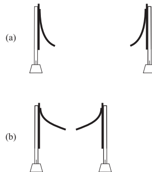
Рис. 7.17: Два электроскопа, наэлектризованные индукцией, получают заряды противоположного знака.
