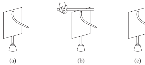
Рис. 6.13: (a) Изначально заряженный электроскоп. (b) Мы держим один конец нейтральной пластиковой соломы в руке, и трогаем край электроскопа другим концом соломы. С полоской ничего не происходит. (c) После удаления соломки, полоса остается в поднятом положении. То есть электризованный электроскоп не разряжается, когда мы трогаем его нейтральной пластиковой соломой.
