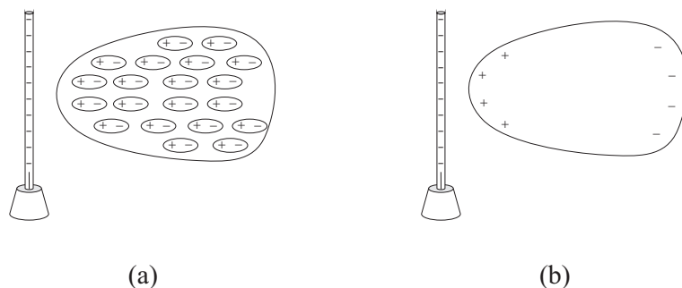
Рис. 7.31: (а) Микроскопическая модель идеализированного изолятора, поляризованного в присутствии другого заряженного тела. (b) Эффективная поляризация диэлектрика в ситуации (а).
