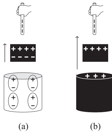
Рис. 8.7: (а) Поляризованный кусок бумаги, который первоначально покоился на изолирующей поверхности, притягивается натертой соломой. (b) Электризованный кусок бумаги, который первоначально лежал на проводящей поверхности, притягивается натертой соломой. Размеры стрелок указывают на интенсивность сил в предположении фиксированного и одинакового расстояния для обоих случаев.
