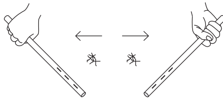
Рис. 5.9: Невозможно объединить два отрицательно заряженных куски хлопка.
