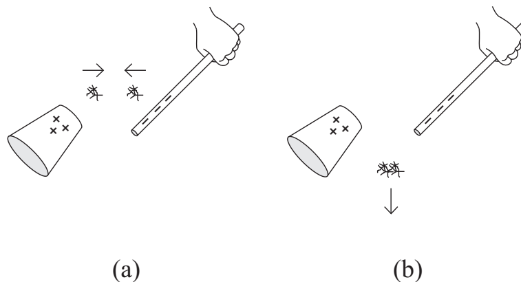
Рис. 5.14: (a) Положительный кусок ваты притягивается отрицательным. (b) После соприкосновения, они падают вместе на землю.
