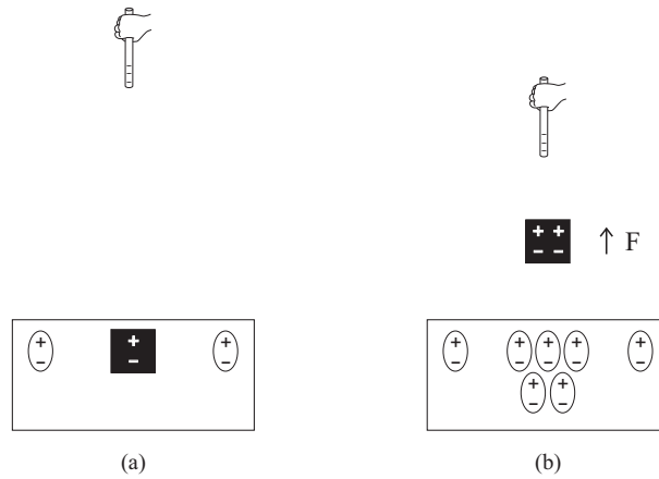
Рис. 8.5: (а) Поляризованный кусочек бумаги поддерживается на поляризованной пенополистироловой пластине в присутствии электризованной соломы, которая находится далеко от бумаги. (б) При перемещении соломы еще ближе к бумаге, мы увеличиваем поляризацию бумаги и пенопласта. Это создает притягивающую бумагу электростатическую силу, которая может превысит вес бумаги. Тогда бумага будет двигаться к соломе.
