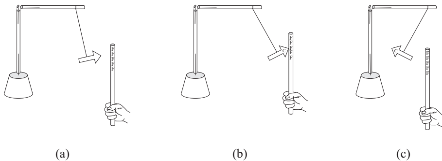
Рис. 4.32: (а) Первоначально стрелка показывает в сторону натертого пластика, так как пластик притягивает ее. (b) Стрелка приходит в контакт с соломкой. (c) После контакта, стрелка отталкивается соломой, кончик стрелки указывает при этом в направлении от соломы.
