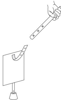
Рис. 6.9: Притяжение между положительной соломой и отрицательным электроскопом.
