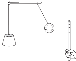
Рис. 8.2: натертая солома поляризует и притягивает бумажный диск.
