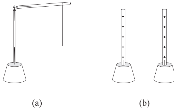
Рис. 5.25: (a) Нить привязана к пластиковой соломе. (b) Противоположно электризованные пластиковые соломки.
