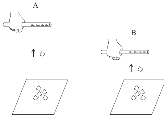
Рис. 5.29: Солома A электризована в большей степени, чем солома B , ибо она начинает притягивать бумажки на большем расстоянии от стола.
