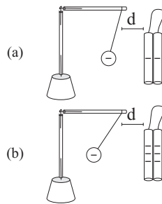
Рис. 5.31: Тела, имеющие разное количество зарядов. Пластики в (b) имеют больший электрический заряд, чем пластики в (a).
