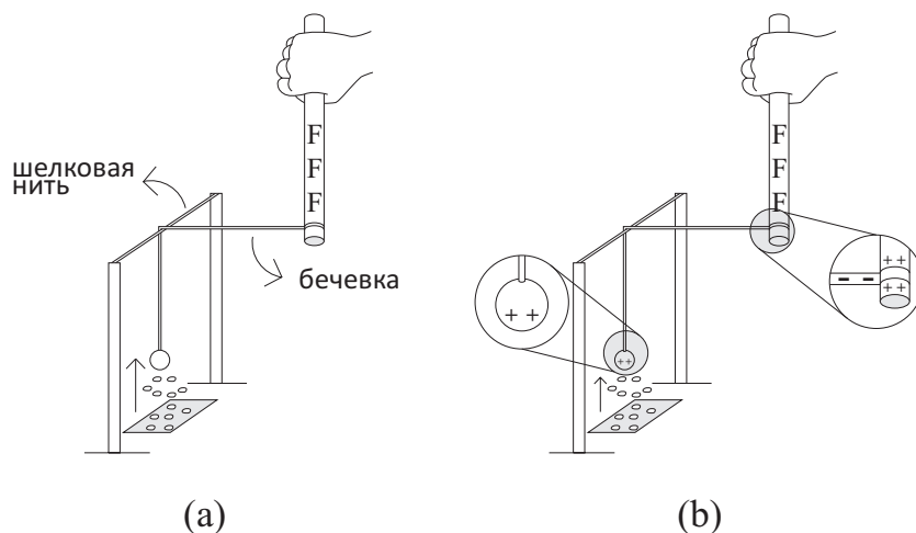
Рис. В.8: (а) Грей наблюдал притяжение латунного листка, когда он натирал стеклянную трубку. В этой ситуации шпагат, прикрепленный к натертой стеклянной трубке, поддерживался шелковой нитью. (b) Схематичное представление зарядов в случае (а).
