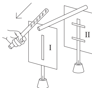
Рис. 6.17: Два изначально разряженных электроскопа с их полосками на внешней стороне. Они соединены между собой нейтральной соломой. Вторая заряженная солома царапает по картону электроскопа I .
