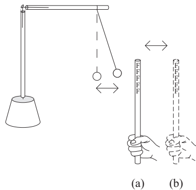
Рис. 4.17: Электрический маятник следует за движением натертого куска пластика. (а) Если солома подносится близко к бумажному диску, диск перемещается к нему. (б) Когда солома удаляется, маятник возвращается в вертикальное положение.
