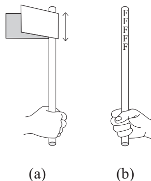
Рис. 2.2: (а) Пластиковая солома, натертая бумагой. (б) Буквой F обозначена натертая область соломы.
