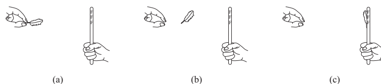
Рис. 4.10: Эксперимент Грея, показывающий притяжение пухового пера натертым стеклом.
