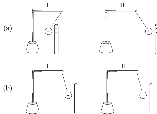
Рис. 5.8: (а) Отрицательное тело (натертая солома) сильно отталкивает другое отрицательное тело (бумажный диск маятника I ), и сильно притягивает положительное тело (бумажный диск маятника II ). (b) Нейтральное тело (ненатертая солома) притягивает положительные и отрицательные тела (бумажные диски маятников I и II ). Кроме того, интенсивность этих сил в случае (а) выше, чем в случае (b).
