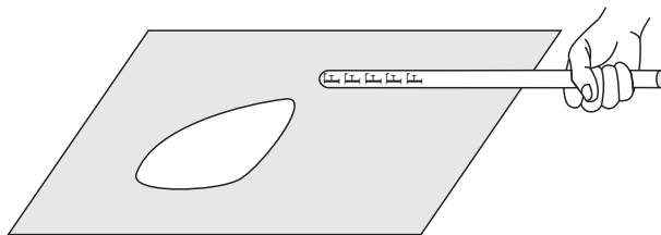
Рис. 2.7: Натертая солома притягивает каплю воды.
