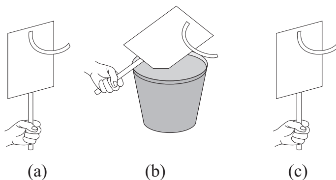
Рис. 6.16: (а) Изначально электризованный электроскоп. (б) Мы погружаем край картона в жидкость. Полоса остается в поднятом состоянии. (с) При удалении электроскопа из жидкости, полоса остается в поднятом состоянии.
