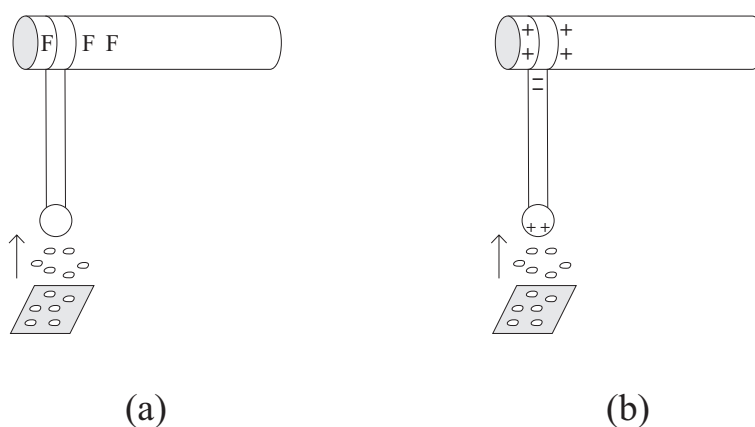
Рис. В.6: (а) Когда Грей натер стеклянную трубку, он обнаружил притяжение легких листочков из латуни телами, прикрепленными к нижнему концу свисающего с трубки шпагата. Притягивающее тело могло быть даже металлическим. (b) Качественное представление зарядов на стекле, наряду с поляризацией шпагата и прикрепленного к нему мяча.
