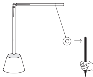
Рис. 4.19: Электрический маятник, который отталкивался натертой соломой после их соприкосновения, теперь притягивается нейтральной деревянной шпажкой.
