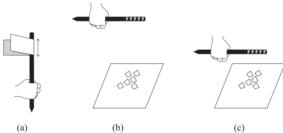
Рис. 2.9: (а) Деревянная шпалка натертая в хлопчатобумажной ткани или шерсти. (в) Натертая шпалка расположена далеко от кусков бумаги. (с) Мы видим, что она не притягивает мелкие куски бумаги, размещенные рядом с ней.
