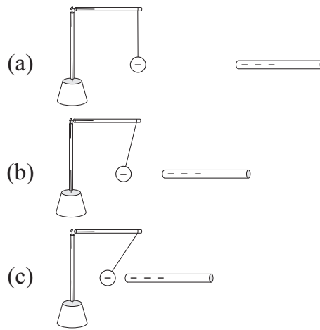
Рис. 5.27: Уменьшая расстояние между отрицательным бумажным диском и отрицательным кончиком натертой соломки, мы увеличиваем силу отталкивания между ними.
