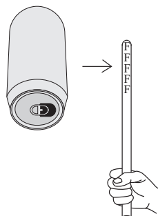
Рис. 2.5: Натертая солома притягивает металлическую банку.
