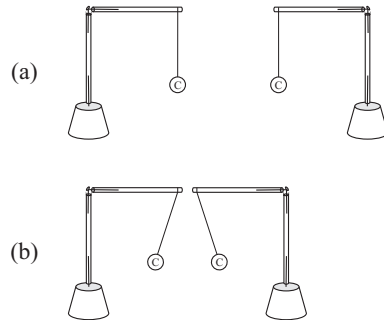
Рис. 4.27: (а) Заряженные маятники висят вертикально, когда они находятся далеко друг от друга. (б) Близко расположенные заряженные маятники отталкивают друг друга.
