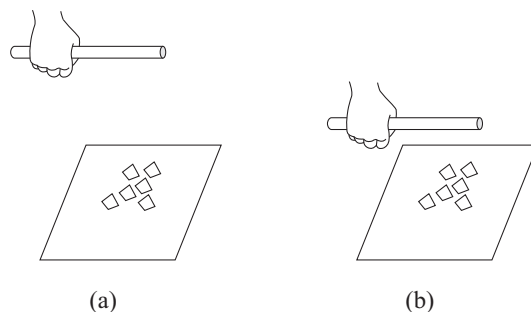
Рис. 2.1: (a) Пластиковая солома далеко от кусочков бумаги. (b) Когда пластиковая солома подносится к кусочкам бумаги, ничего не происходит с ними.
