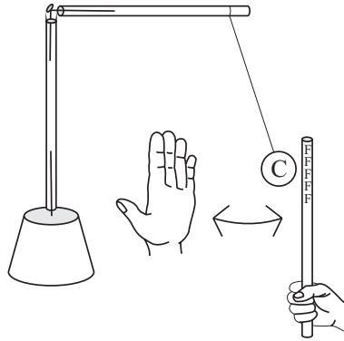
Рис. 4.26: Маятник колеблется между натертой пластиковой соломой и рукой, касаясь каждую из них.
