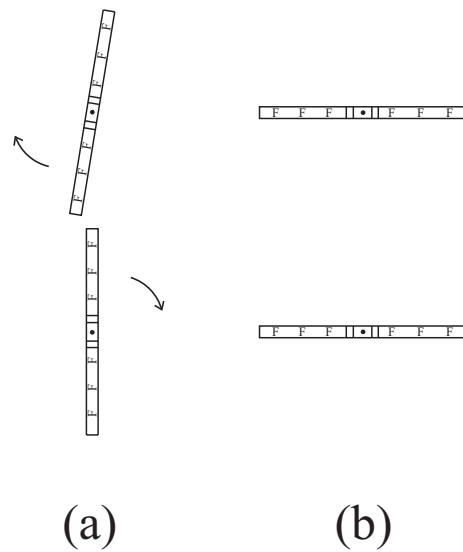
Рис. 4.3: (а) Отталкивание между двумя пластиковыми версориумами (вид сверху), которые были натерты по всей их длине, когда они размещены рядом и ориентированы в одном направлении. (b) Конечные равновесные ориентации двух версориумов.
