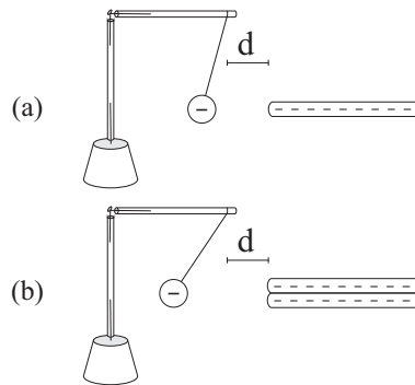
Рис. 5.30: (а) Сила, оказываемая заряженной соломой на заряженный маятник, меньше, чем (b) сила, действующая на тот же маятник со стороны двух одинаково заряженных соломинок на том же расстоянии от вертикали, проходящей через точку подвеса нити.
