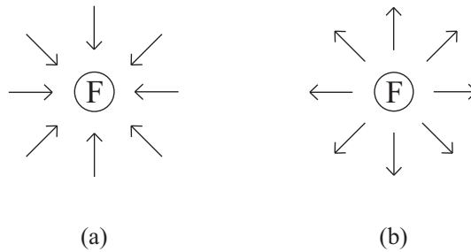
Рис. 4.33: (a) Перед контактом стрелки указывают к натертой соломе, будучи притянутыми к ней. (b) После контакта они указывают в направлении от пластика, отталкиваясь от него.
