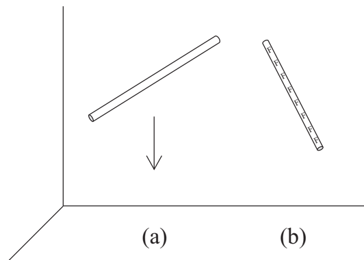
Рис. 3.16: (a) Нейтральная пластиковая солома падает на землю после высвобождения. (b) Пластиковая солома, натертая по всей длине, не падает после высвобождения и держится на стене.
