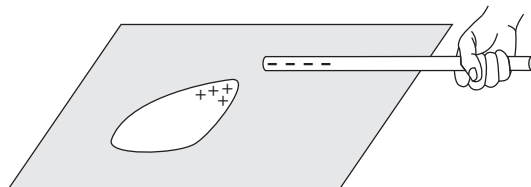
Рис. 7.36: Электрические заряды на капле воды, находящейся рядом с натертой пластиковой соломой.
