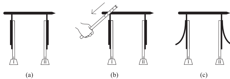
Рис. 6.20: (а) Два первоначально разряженных электроскопа соединены деревянным шпательком. (b) Мы царапаем только электроскоп I наэлектризованной соломой. (с) Электризованная солома удаляется. Мы видим, что оба электроскопа получили заряд.
