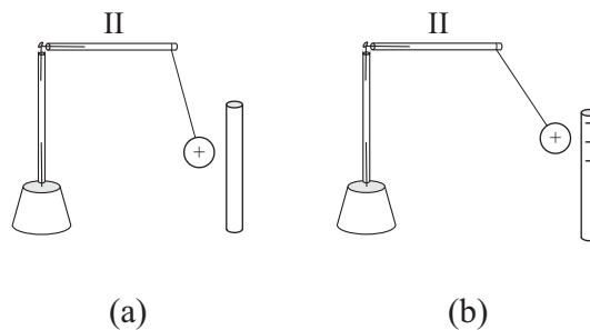
Рис. 5.6: Притяжение между положительным маятником и нейтральной соломой, (а), меньше притяжения между положительным маятником и отрицательной соломой, (b).
