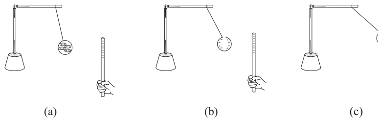
Рис. 8.4: (a) Поляризованный изолятор притягивается близлежащим заряженным телом. (b) Притяжение поляризованного проводника. (c) Притяжение заряженного проводника. Сила растет от (a) до (c), натертая солома находится при этом на одном и том же расстоянии от электрических маятников.
