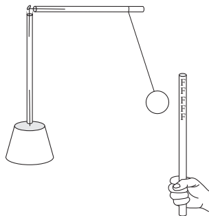
Рис. 4.16: Натертый пластик притягивает бумажный диск расположенного рядом электрического маятника.
