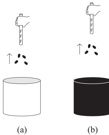
Рис. 7.45: (а) Кусочки бумаги на изолирующей поверхности притягиваются натертой соломой. (b) Кусочки бумаги на проводящей поверхности притягиваются натертой соломой. Минимальное расстояние, на котором солома может притянуть бумажки, больше в случае (b), чем в случае (a). Стрелки указывают направление движения.
