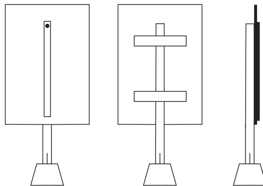
Рис. 6.2: (а) Вид электроскопа спереди. (b) Вид сзади. (с) Вид сбоку.
